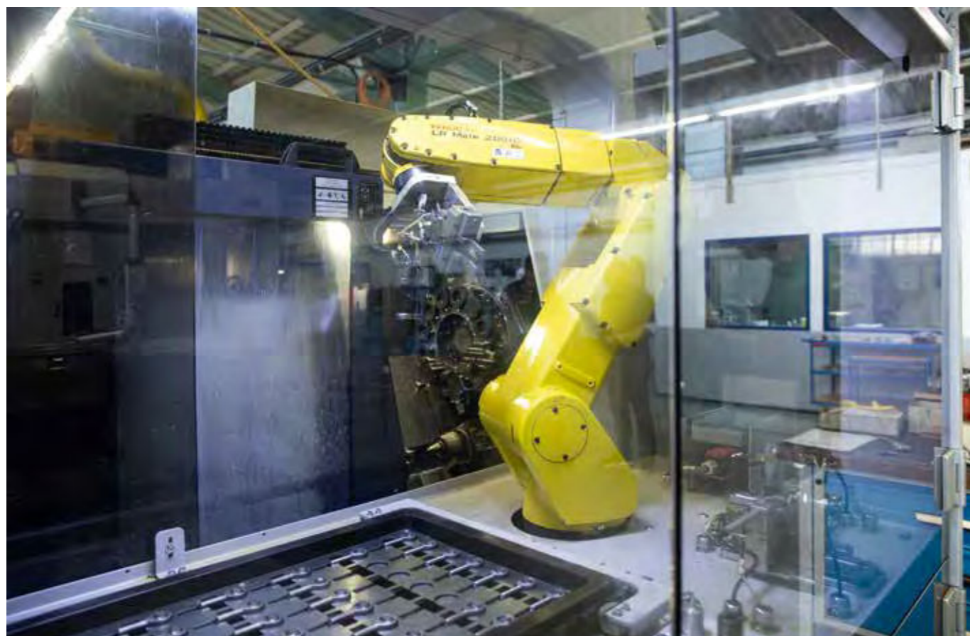
Hi-Tech Produktion bei Durbal Hi-Tech production at Durbal
